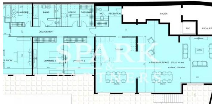
PLAN R+5 LE 29.09.1 avenue Varravilla ROQUEBRUNE CAP MA
